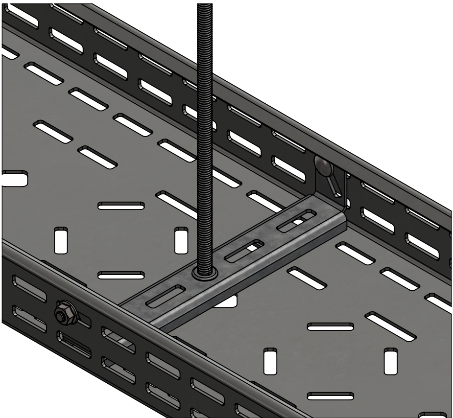
Przykład montażu:
