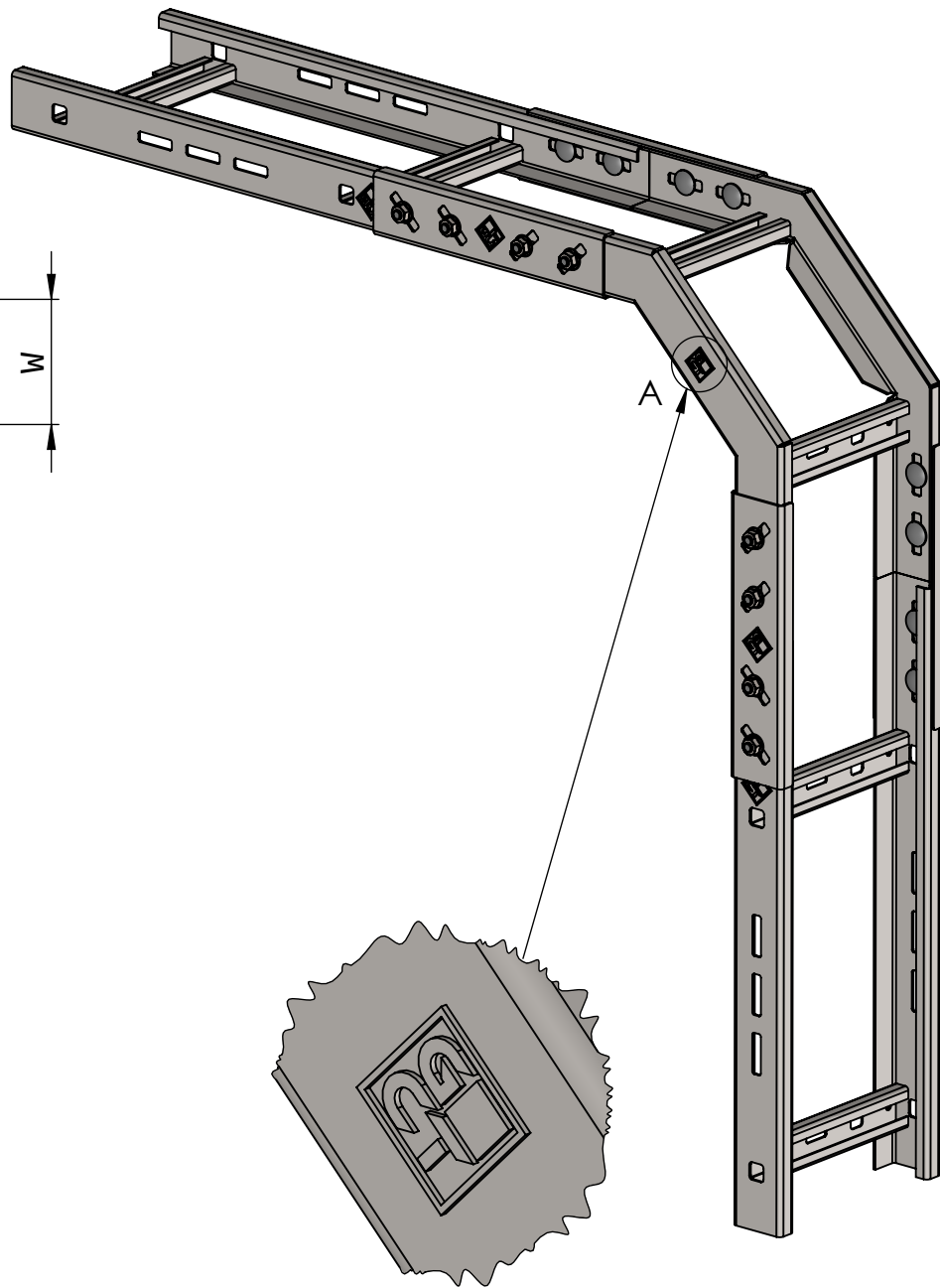
Przykład montażu:
