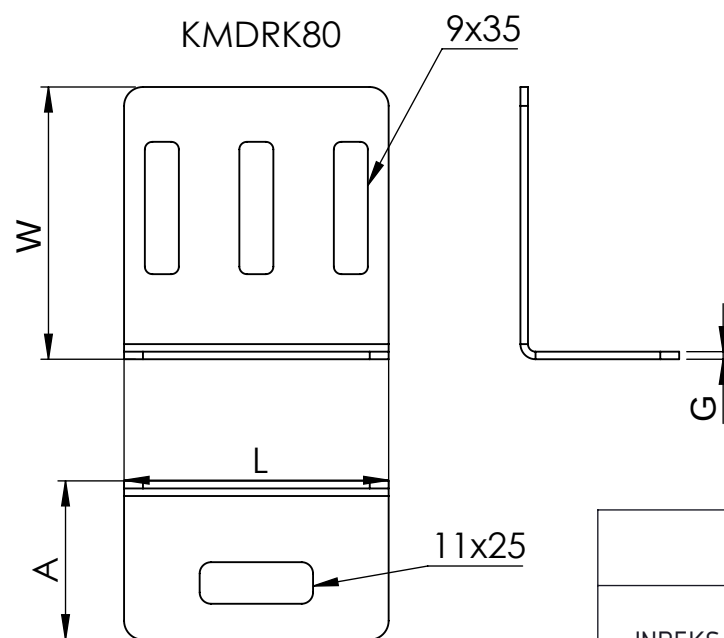
Kątownik montażowy drabiny kablowej - KMDRK-2,0
