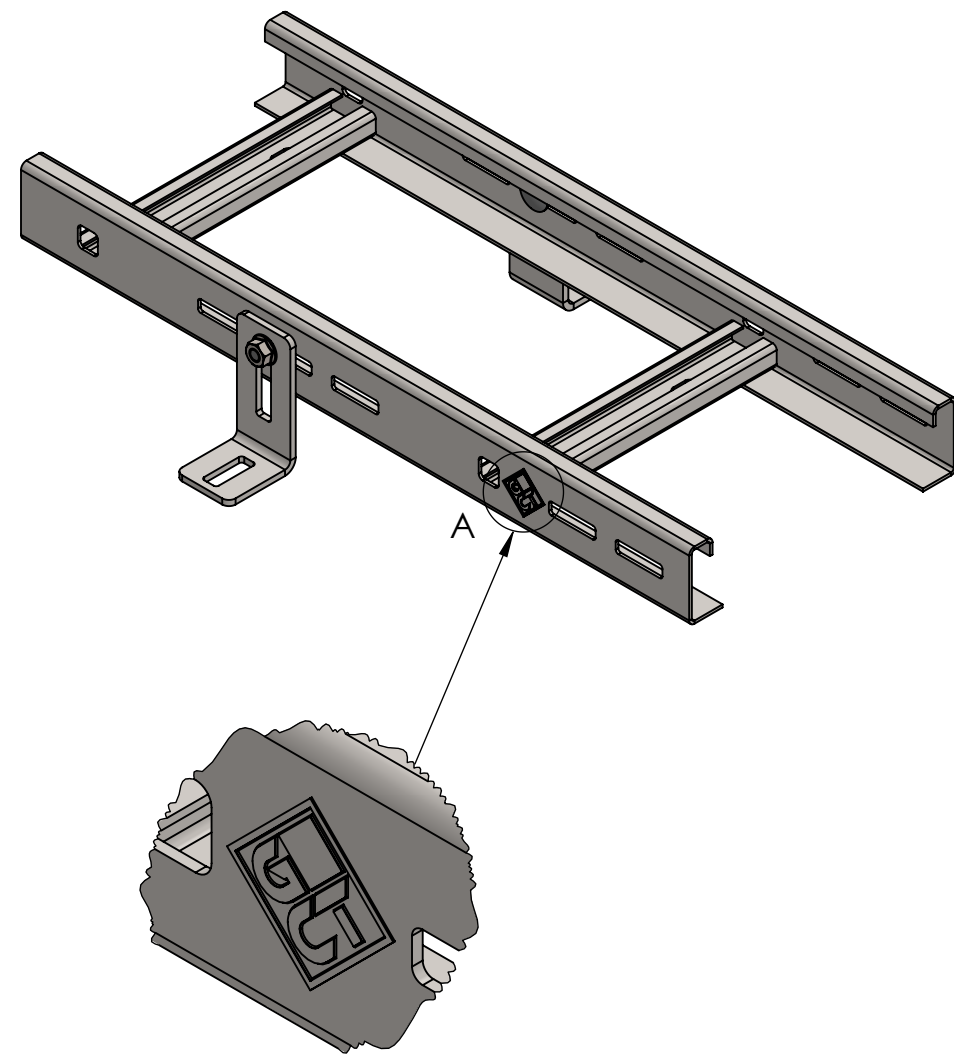
Przykład montażu:
