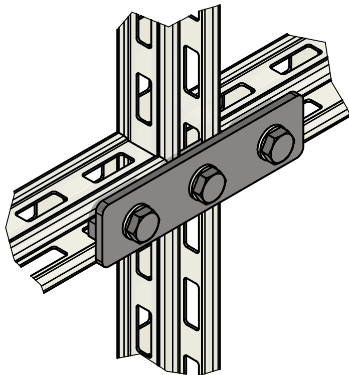
Przykład montażu:
